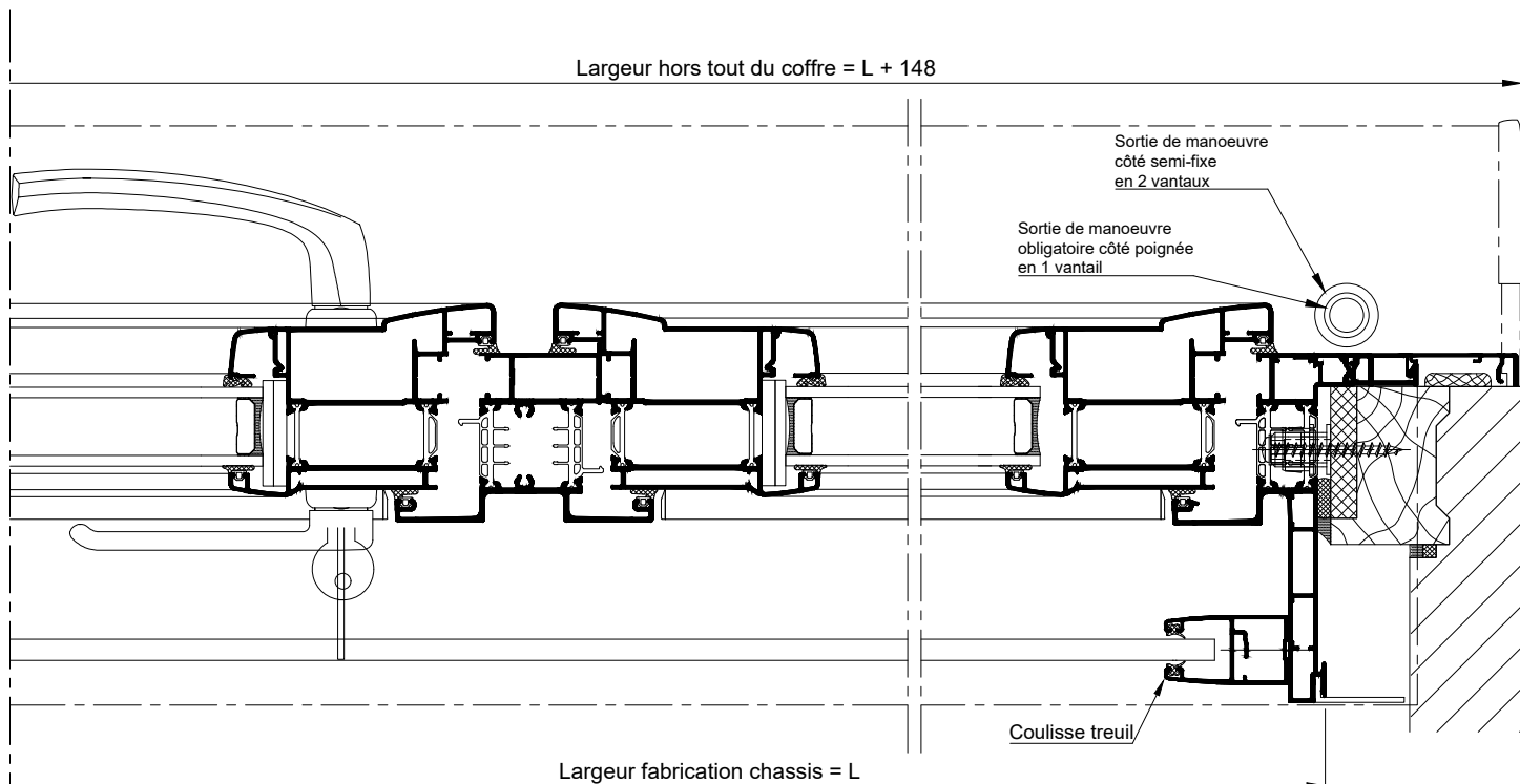
COUPE HORIZONTALE PARTIELLE Ech 1/3
