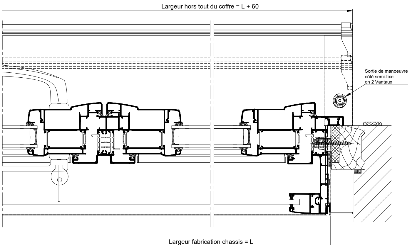
COUPES HORIZONTALES Ech 1/3
