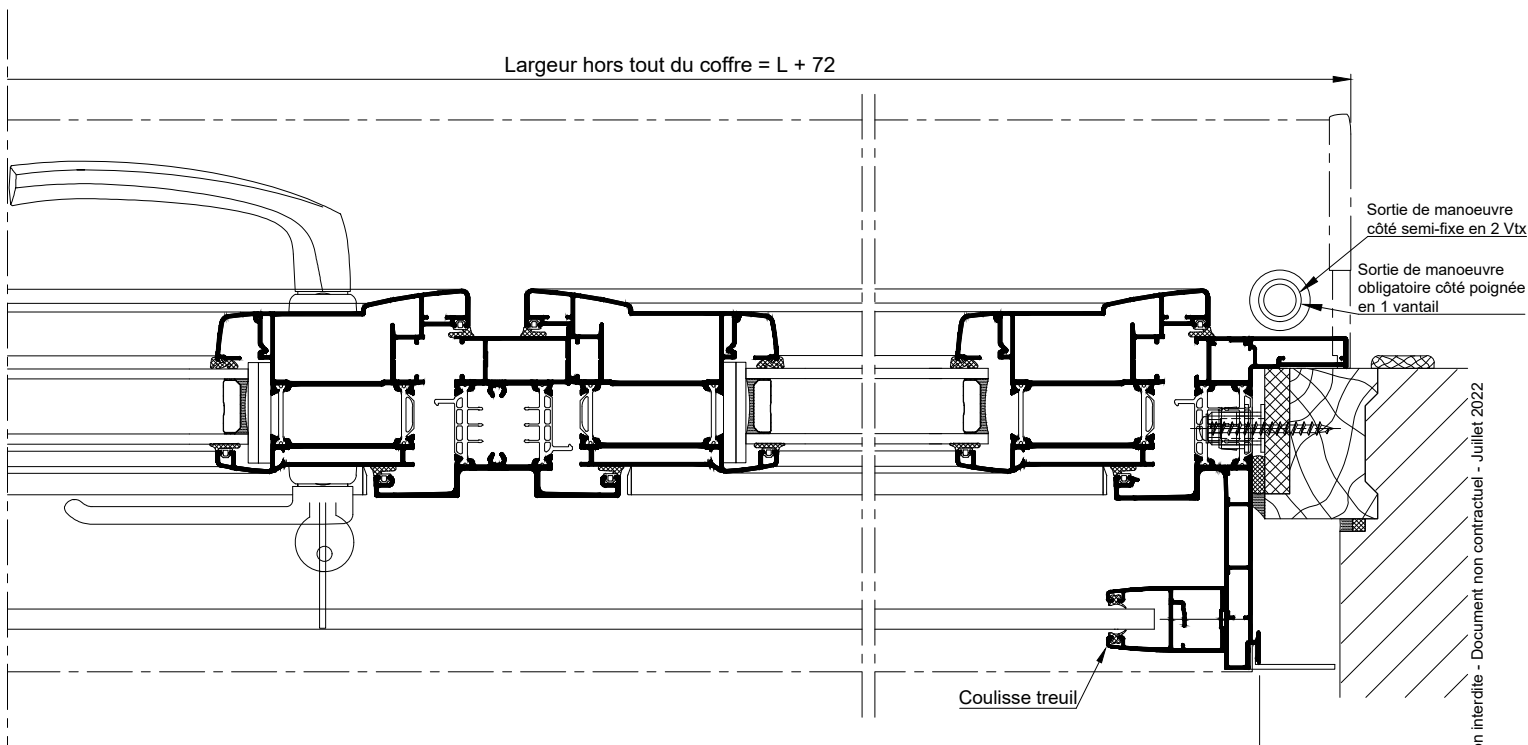
COUPE HORIZONTALE PARTIELLE Ech 1/3
