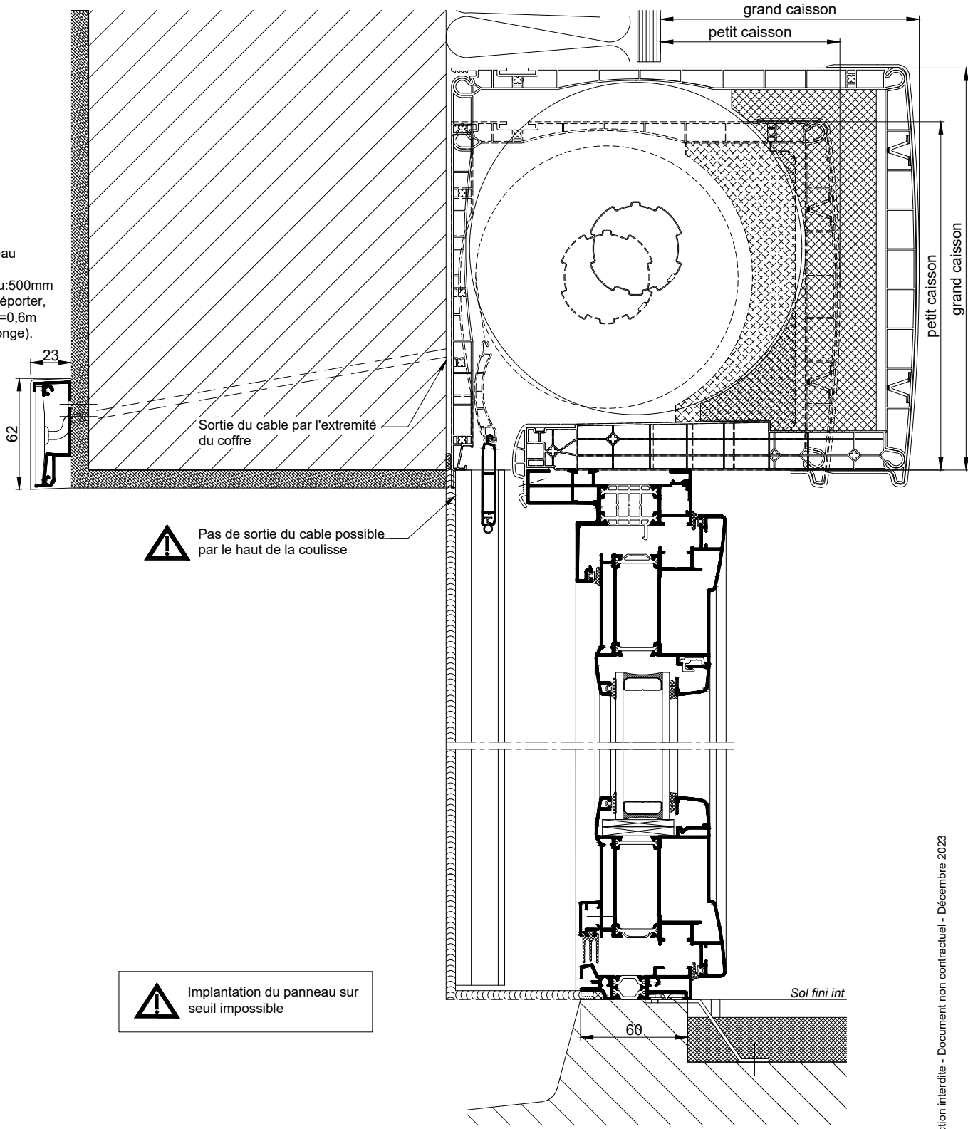
COUPE VERTICALE Ech 1/3
