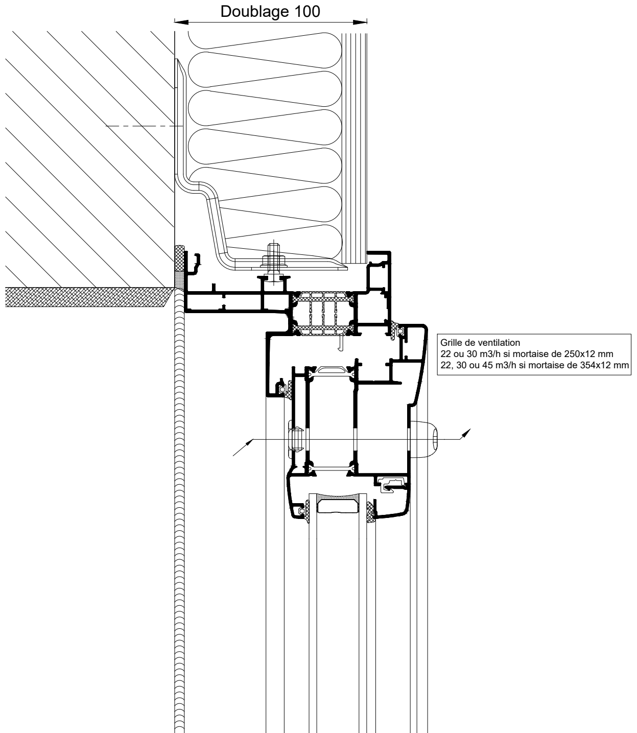
COUPE VERTICALE Ech 1/3
