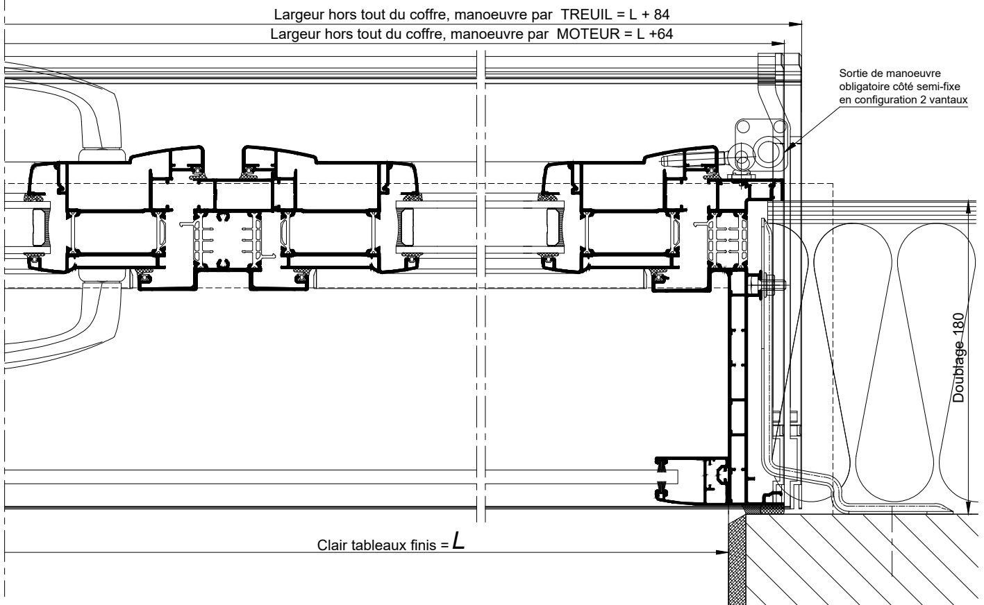
COUPES HORIZONTALES Ech 1/3
