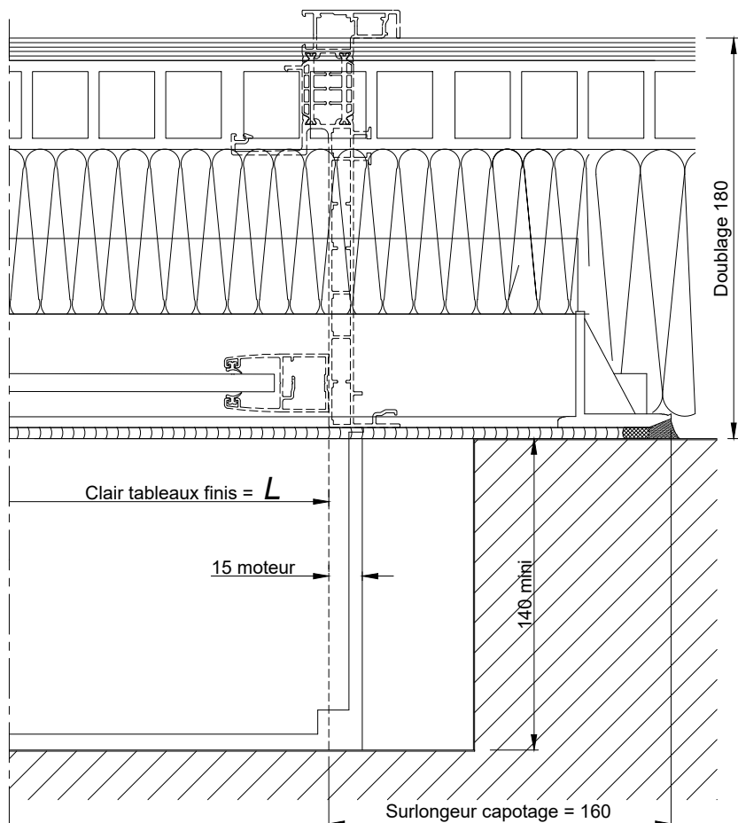
COUPE HORIZONTALE PARTIELLE Ech 1/3
