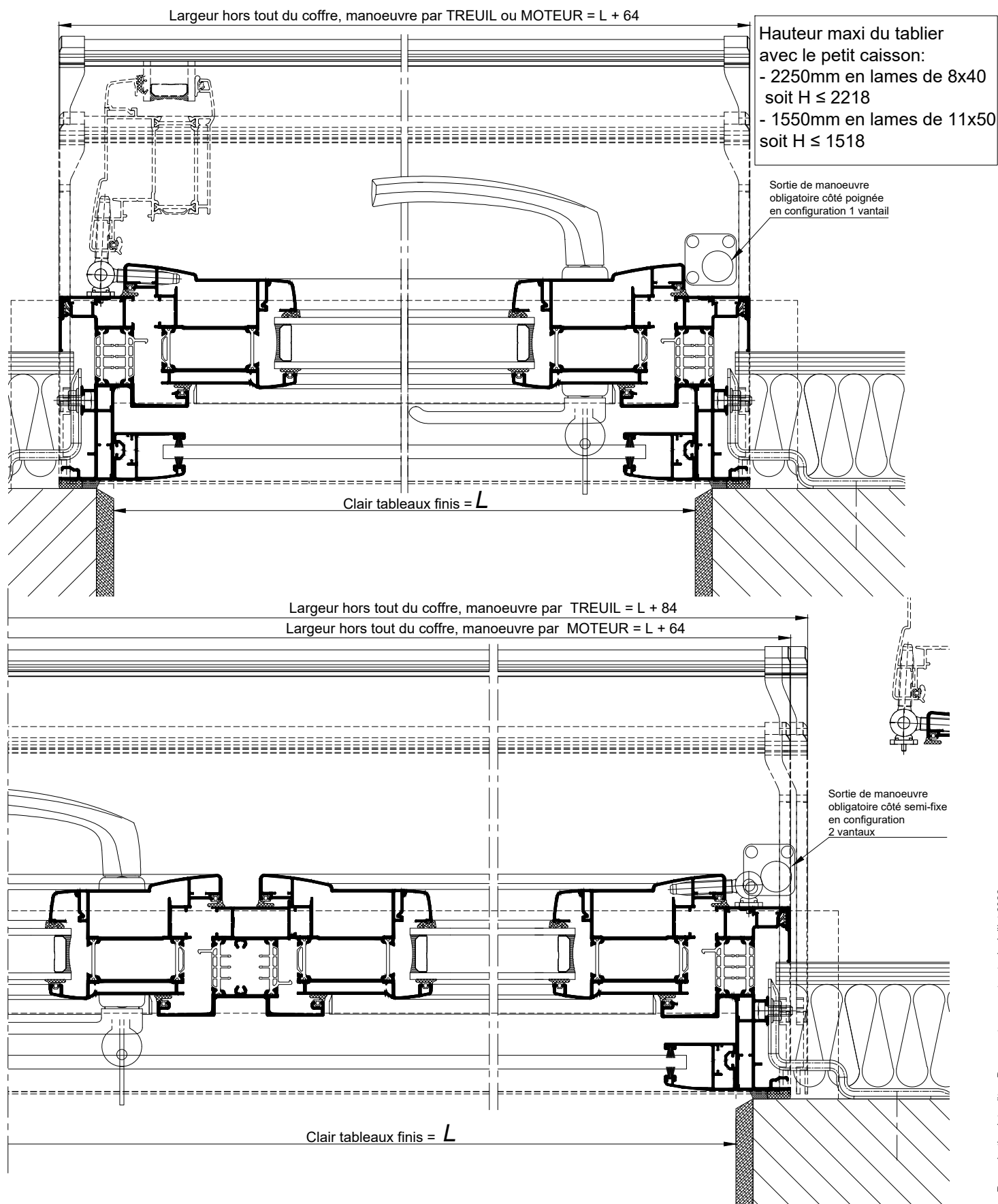
COUPES HORIZONTALES Ech 1/3
