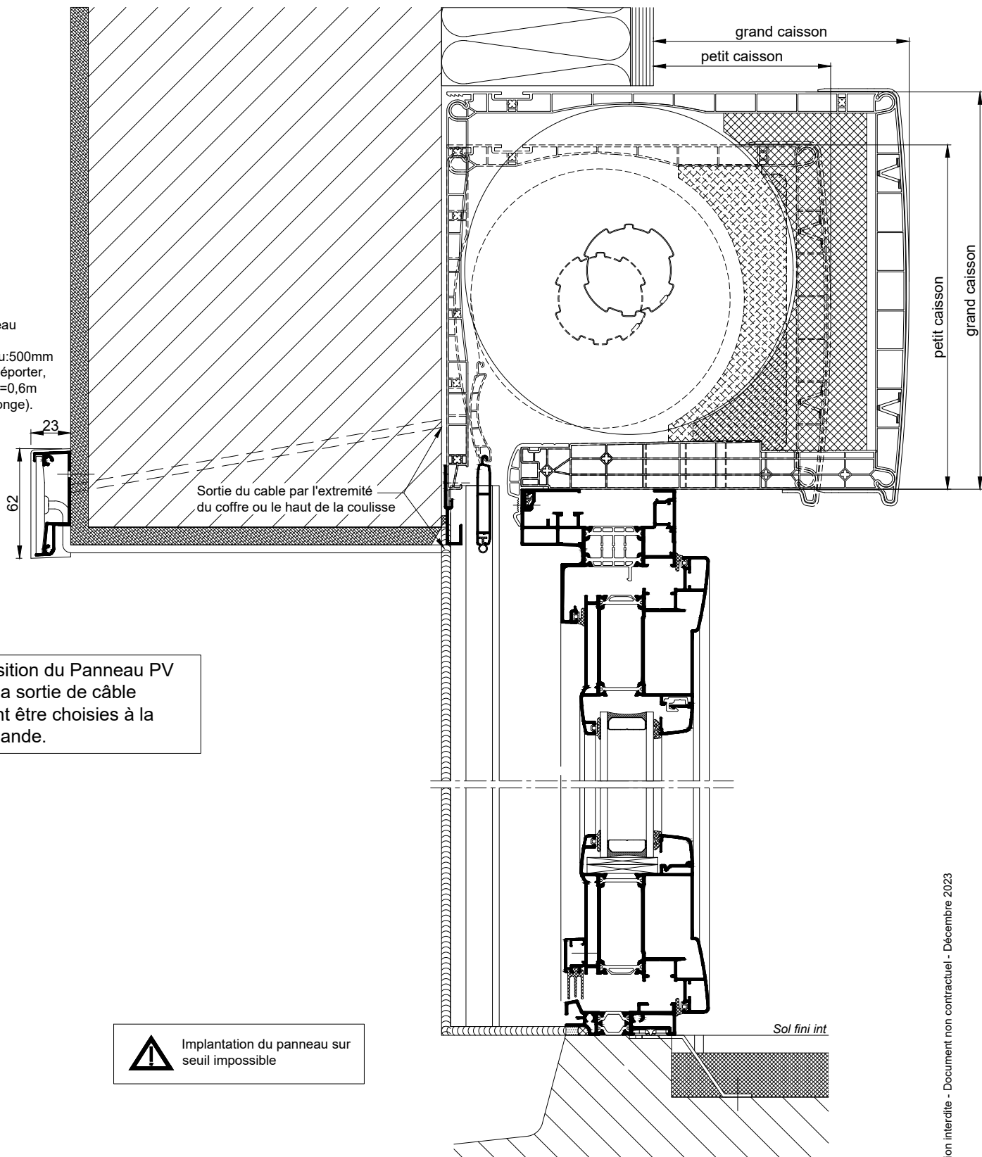
COUPE VERTICALE Ech 1/3
