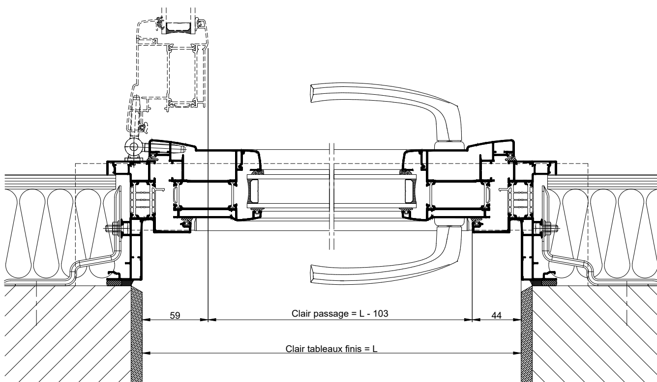
COUPE HORIZONTALE Ech 1/3
