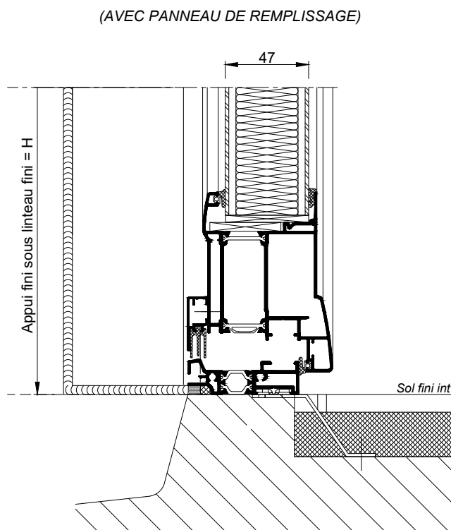
COUPE VERTICALE PARTIELLE Ech 1/3
