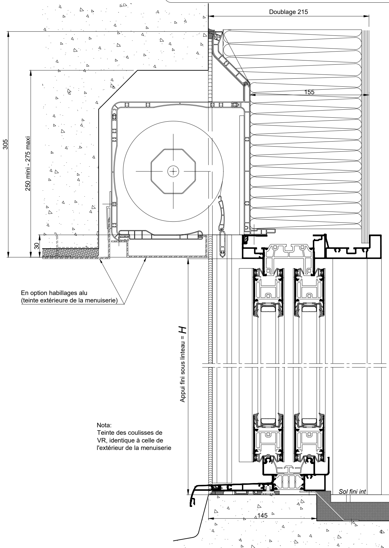
COUPE VERTICALE Ech 1/3
