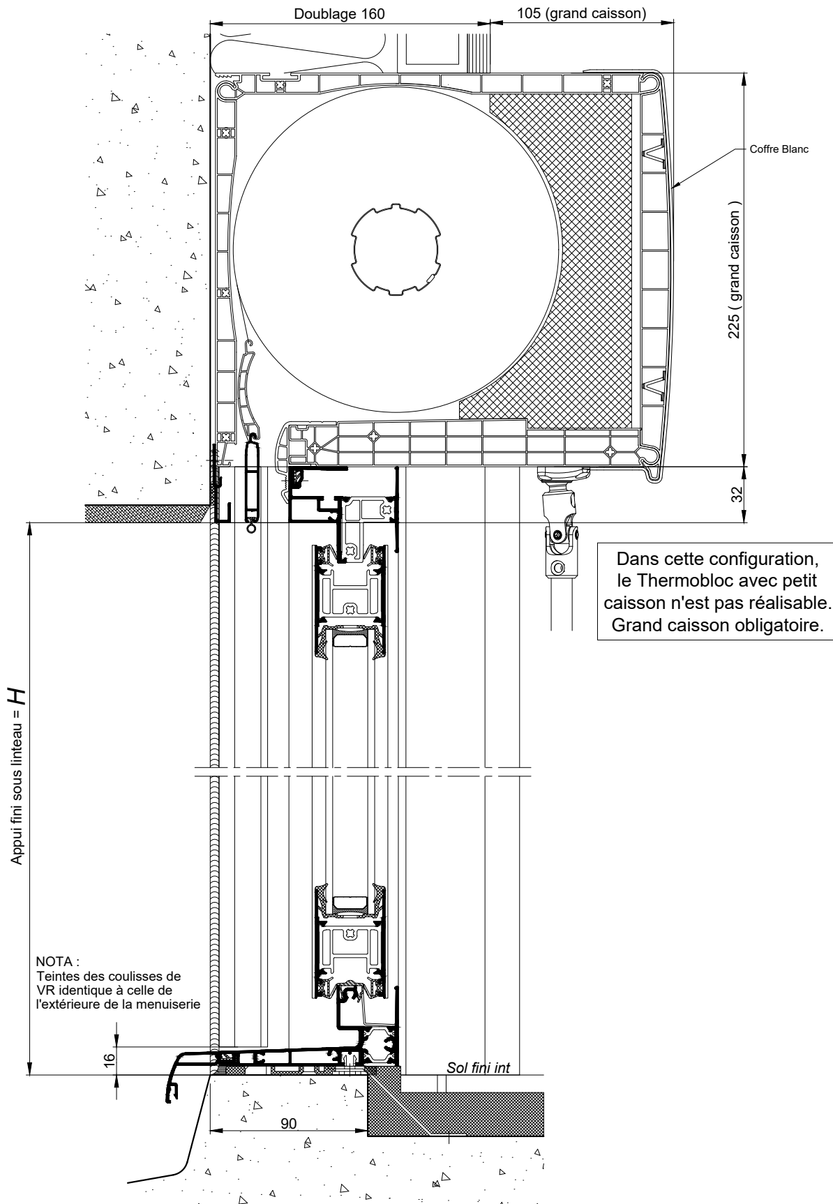
COUPES VERTICALES Ech 1/3
