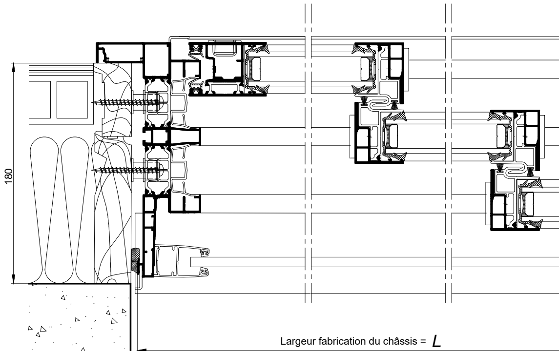
COUPE HORIZONTALE Ech 1/3
