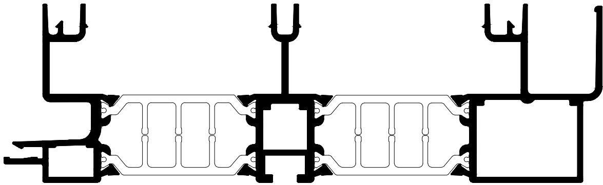
Pose n°7 et option traverse basse sans aile
