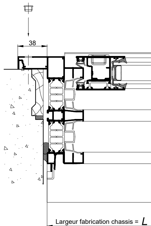
COUPE HORIZONTALE PARTIELLE Ech 1/3
