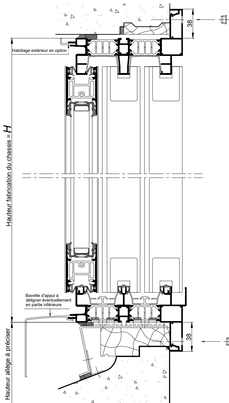
COUPE VERTICALE Ech 1/3
