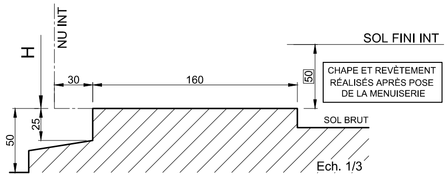
DETAIL : ENCASTREMENT DE 50 MM (VALABLE ÉGALEMENT POUR PASSAGE HANDICAPÉ)
