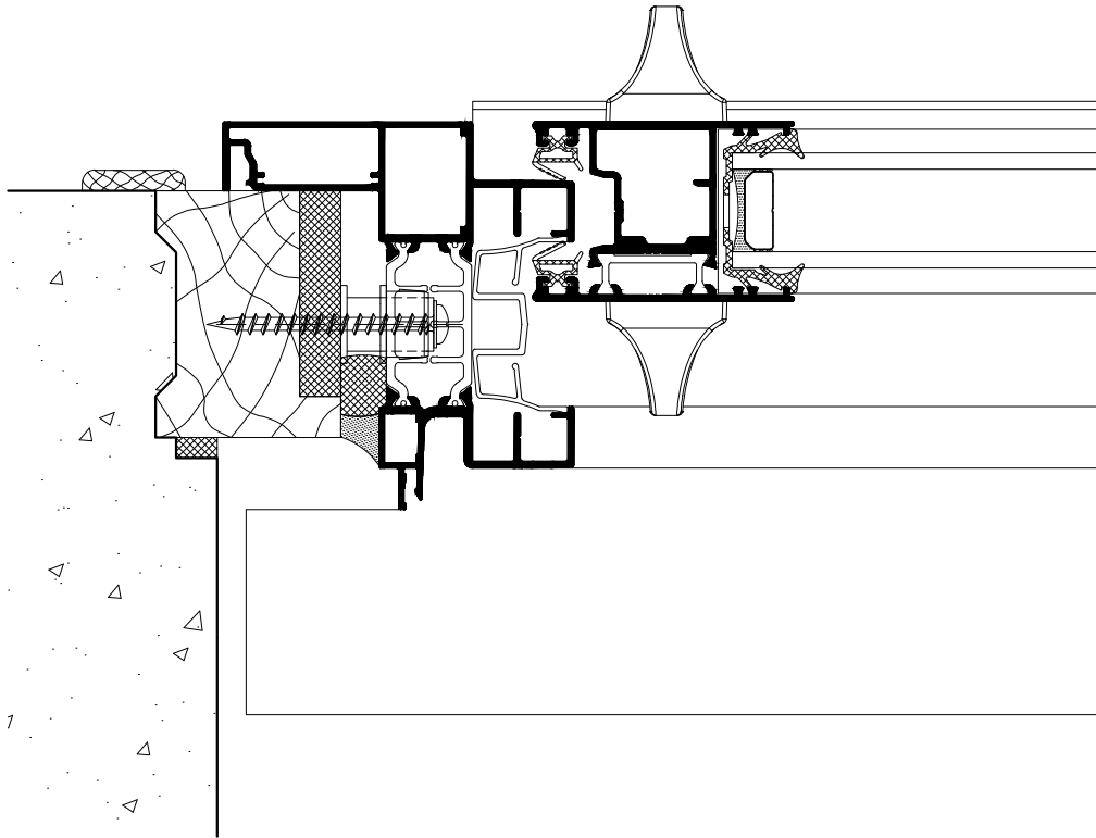
COUPE HORIZONTALE PARTIELLE
