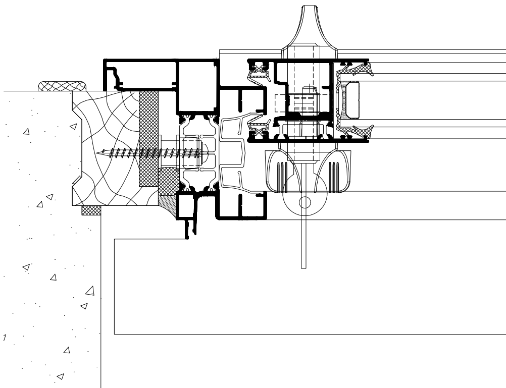
COUPE HORIZONTALE PARTIELLE Ech 1/2
