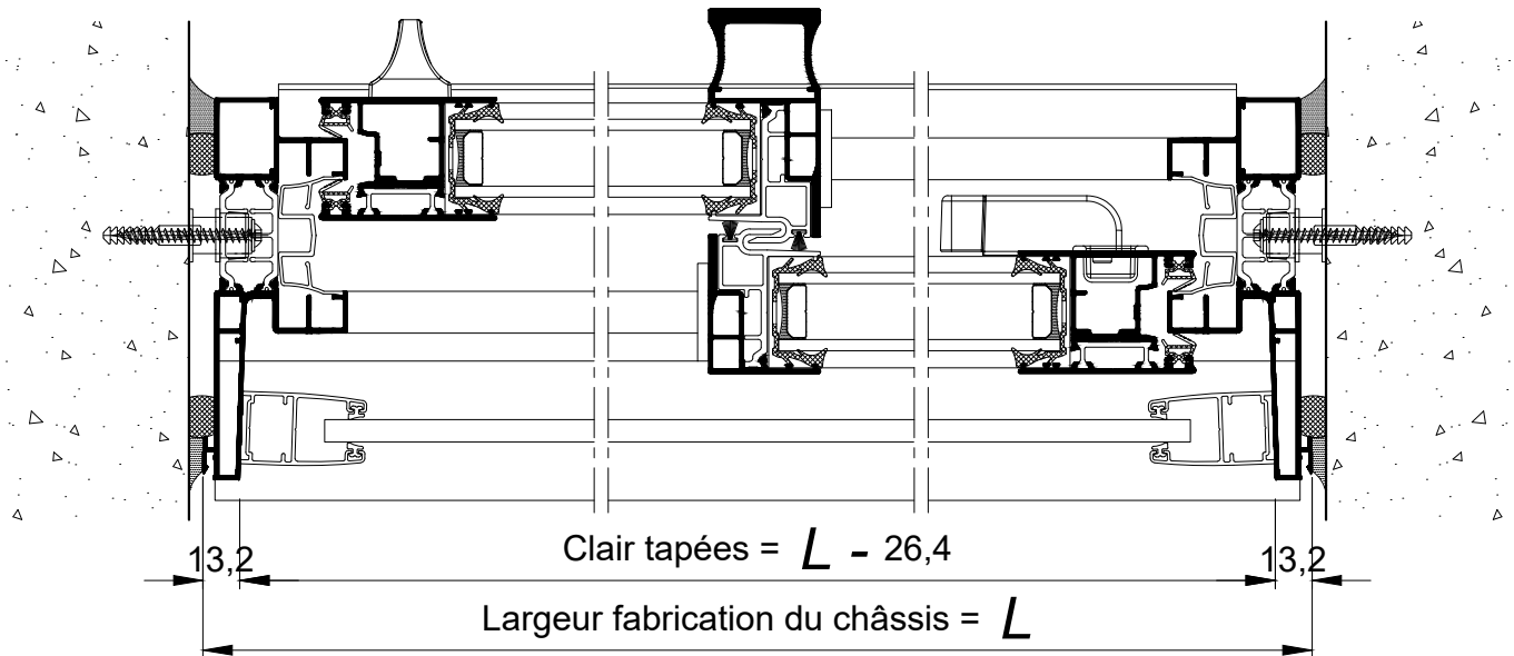
COUPE HORIZONTALE Ech 1/3
