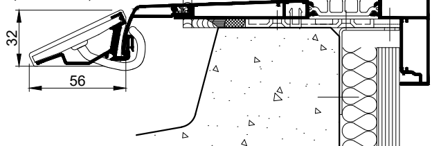
COUPE VERTICALE Ech 1/3
