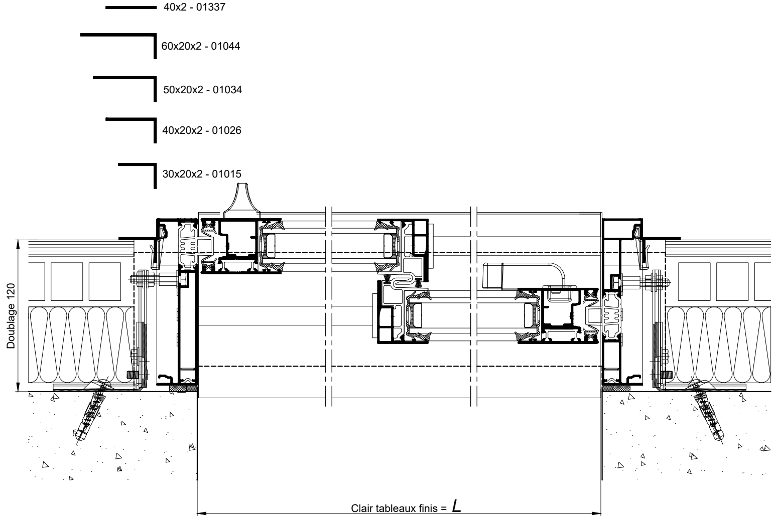
COUPE VERTICALE Ech 1/3
