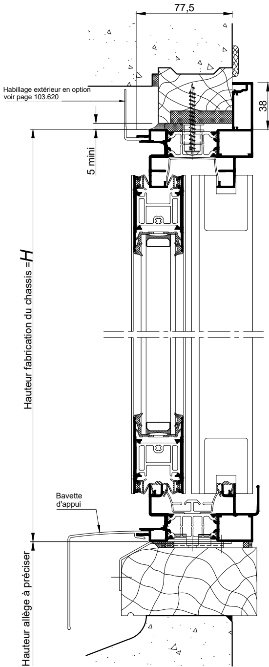
COUPE VERTICALE Ech 1/3
