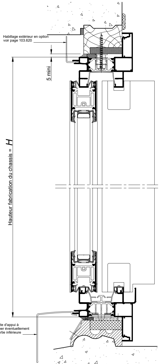
COUPES 1-1 VERTICALES Ech 1/3
