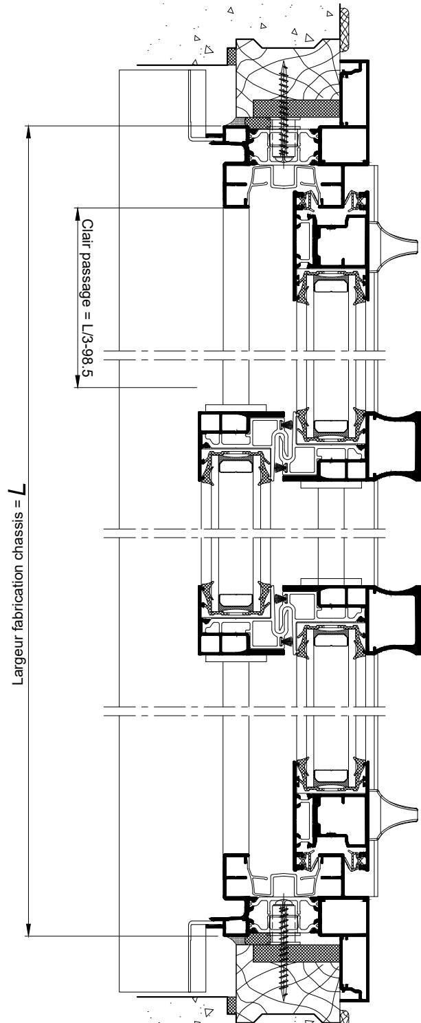
COUPE 2-2 HORIZONTALE Ech 1/3
