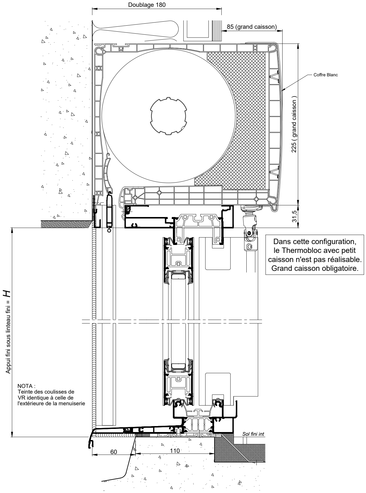
COUPE VERTICALE Ech 1/3
