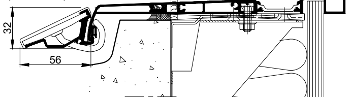
COUPE VERTICALE Ech 1/3
