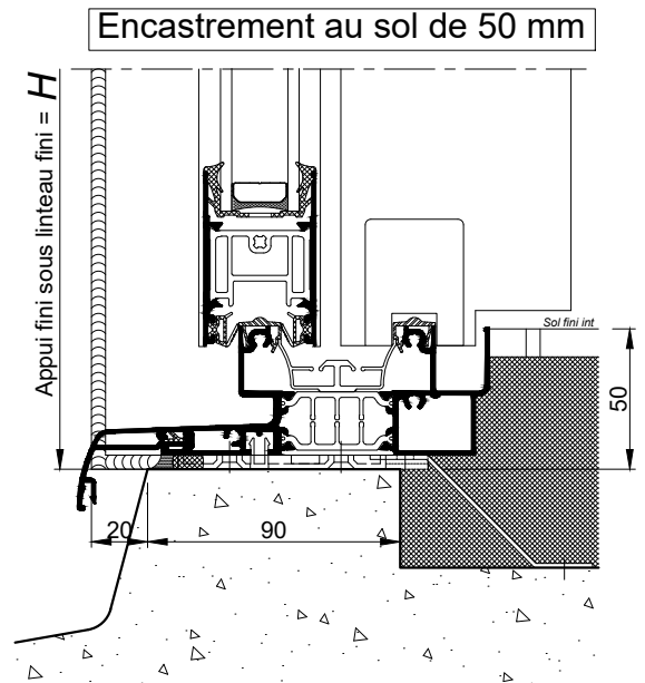
COUPE VERTICALE PARTIELLE Ech 1/3
