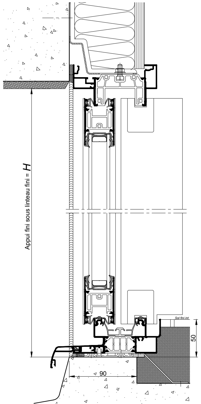
COUPES VERTICALES Ech 1/3
