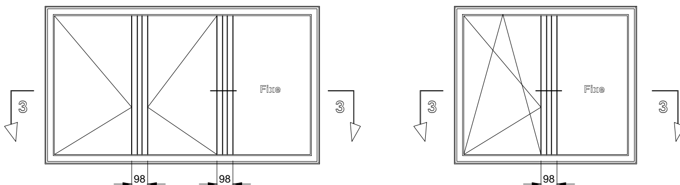
Elévation extérieure
