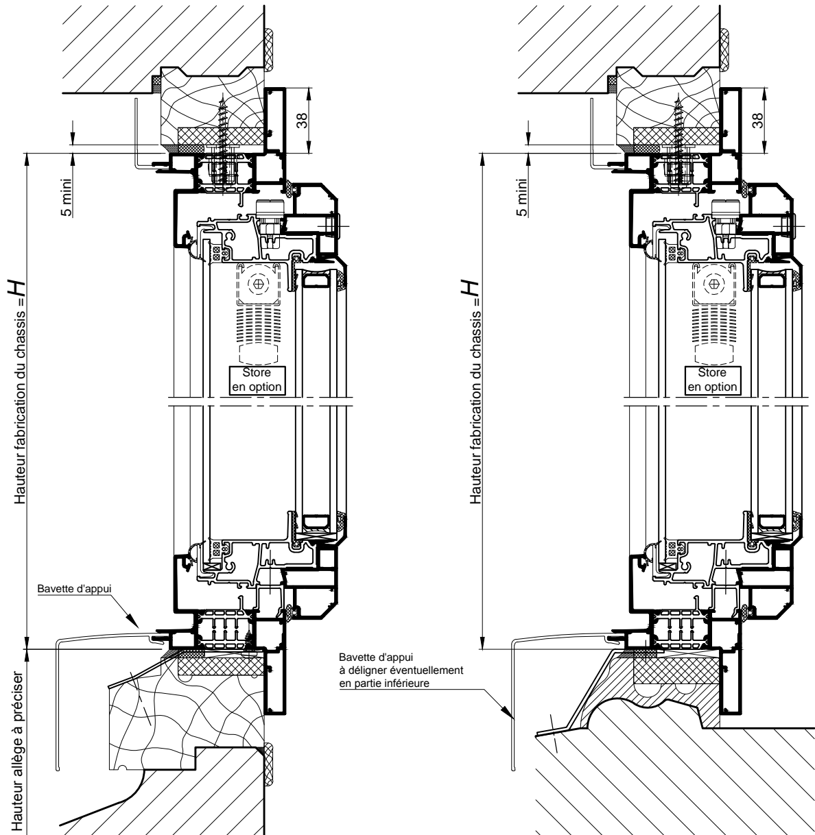
COUPE VERTICALE Ech 1/3
