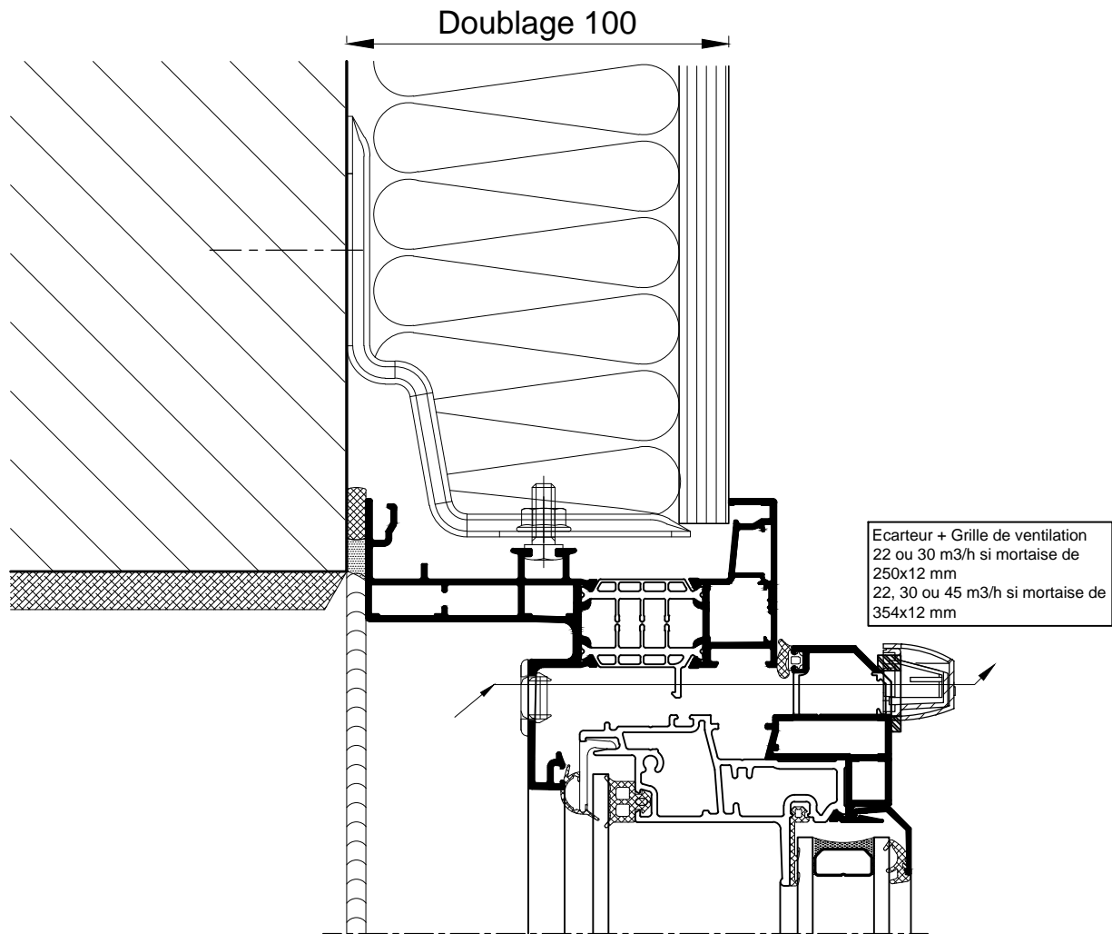
COUPE VERTICALE PARTIELLE Ech 1/2
