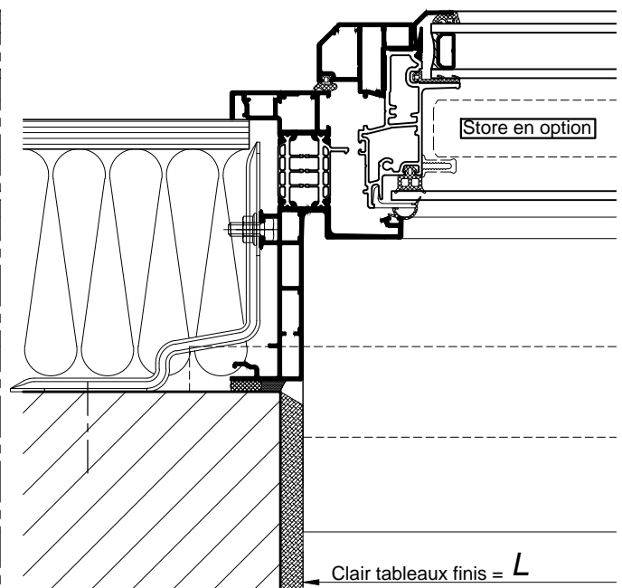
COUPE HORIZONTALE Ech 1/3
