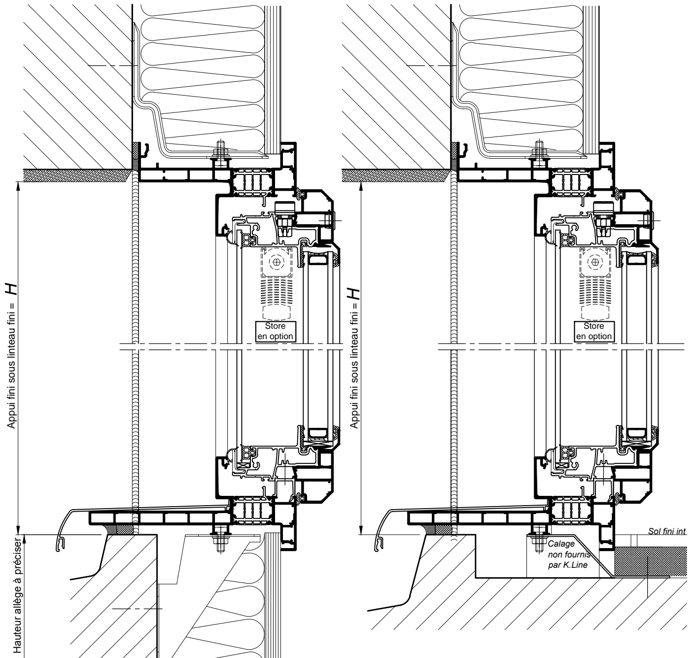
COUPE VERTICALE Ech 1/3
