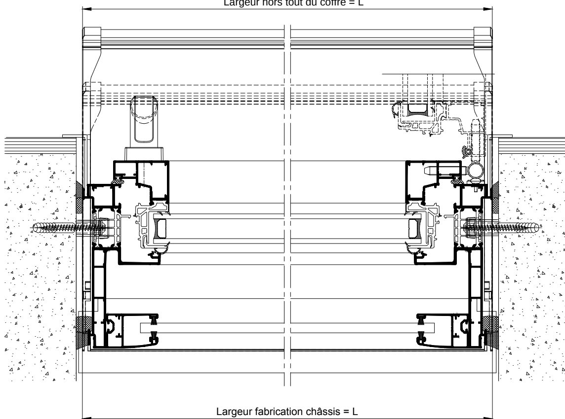
COUPE HORIZONTALE Ech 1/3
