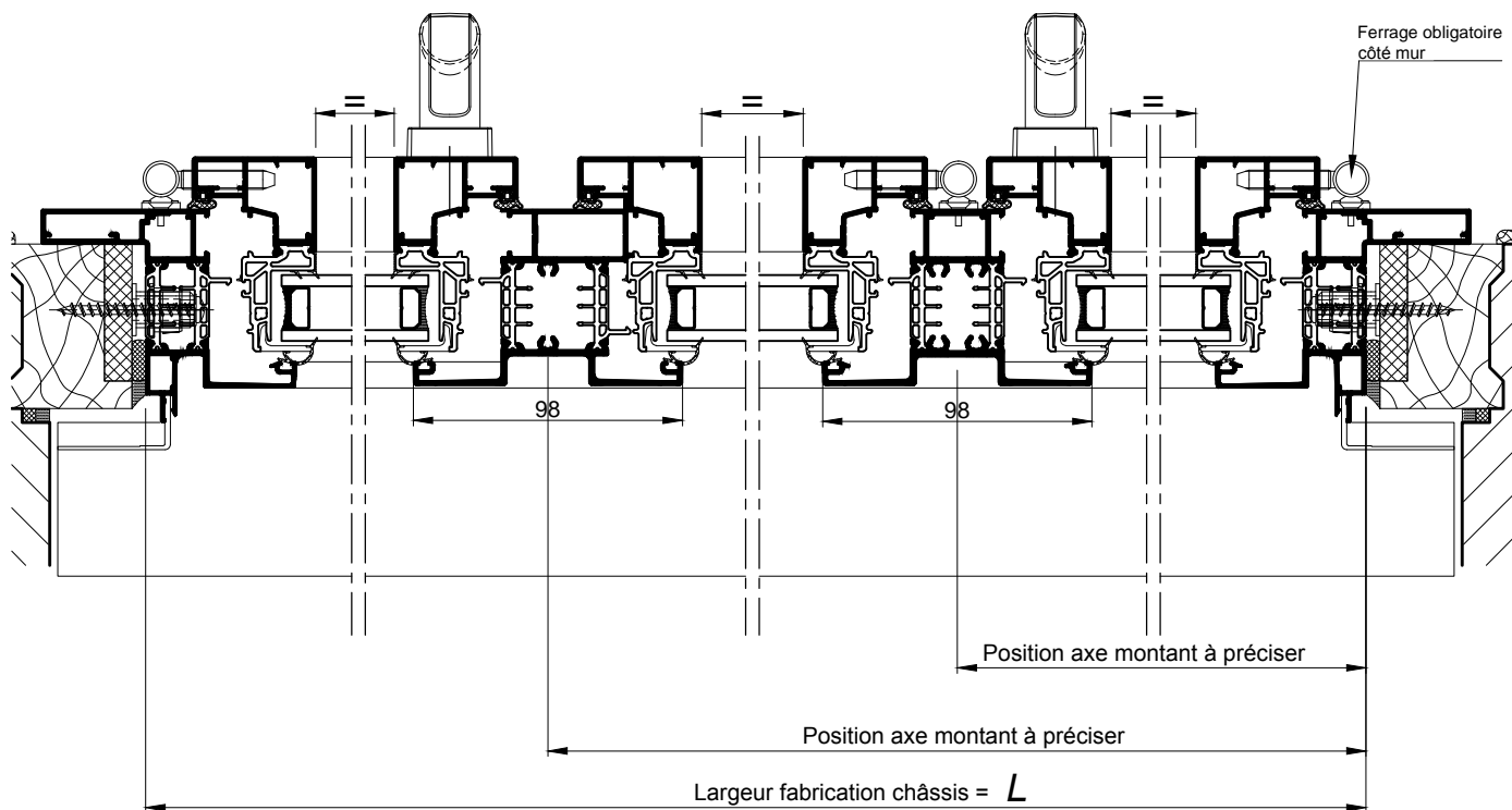
COUPE 3-3 HORIZONTALE Ech 1/3
