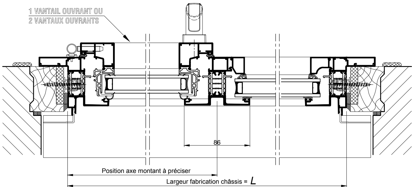
COUPE 3-3 HORIZONTALE Ech 1/3
