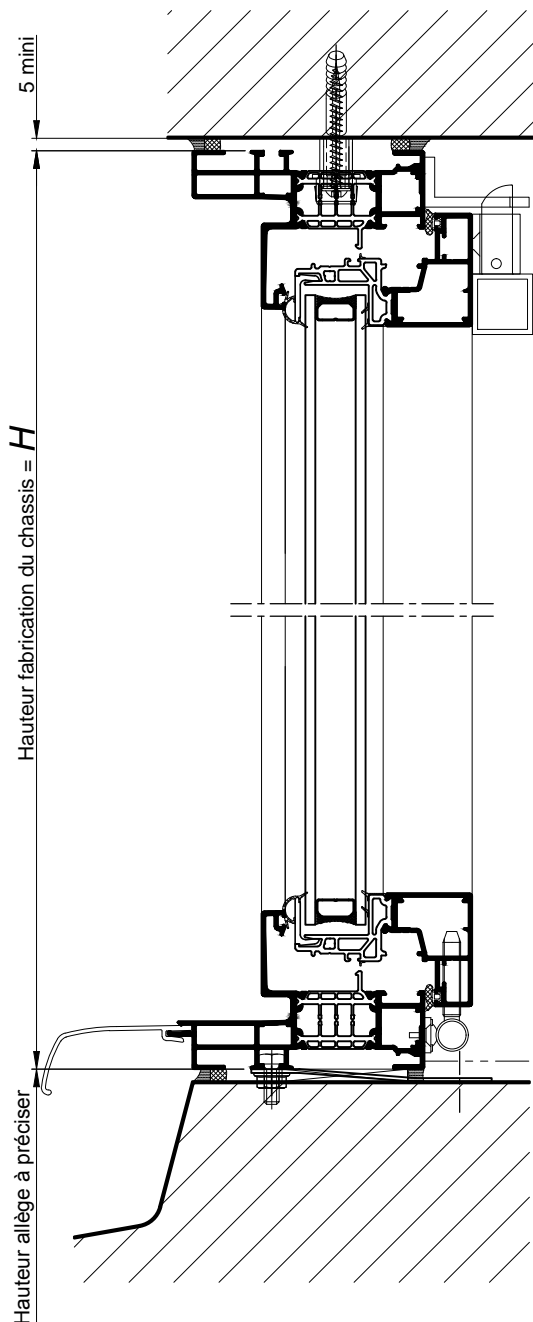
COUPE VERTICALE Ech 1/3
