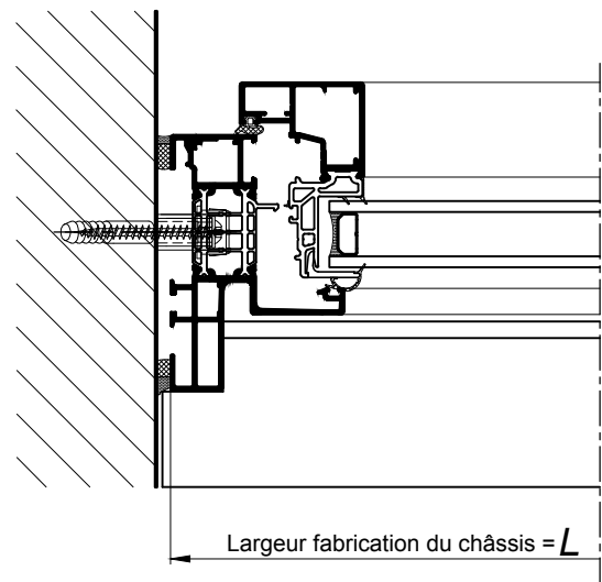
COUPE HORIZONTALE PARTIELLE Ech 1/3
