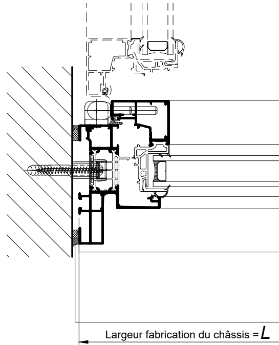
COUPE HORIZONTALE PARTIELLE Ech 1/3
