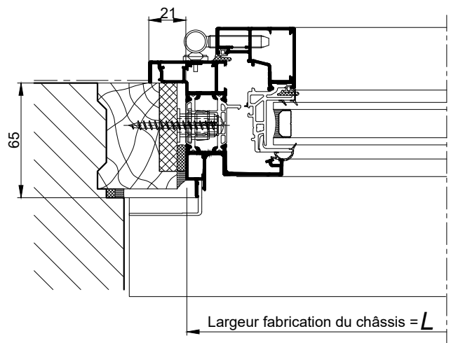
COUPE HORIZONTALE PARTIELLE Ech 1/3
