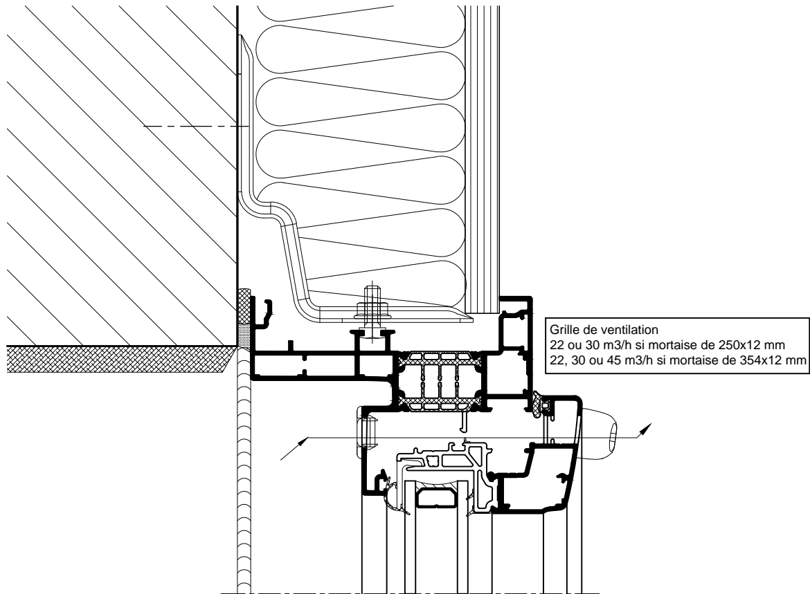
COUPE VERTICALE PARTIELLE Ech 1/2
