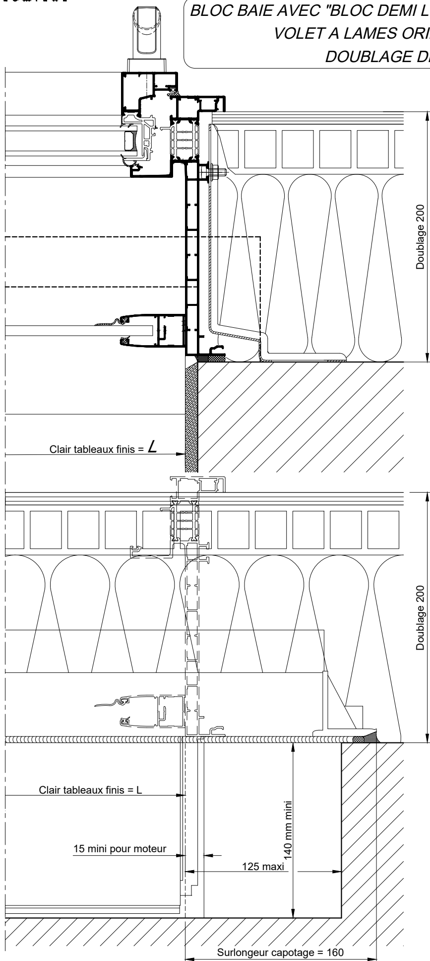
COUPES HORIZONTALES Ech 1/3
