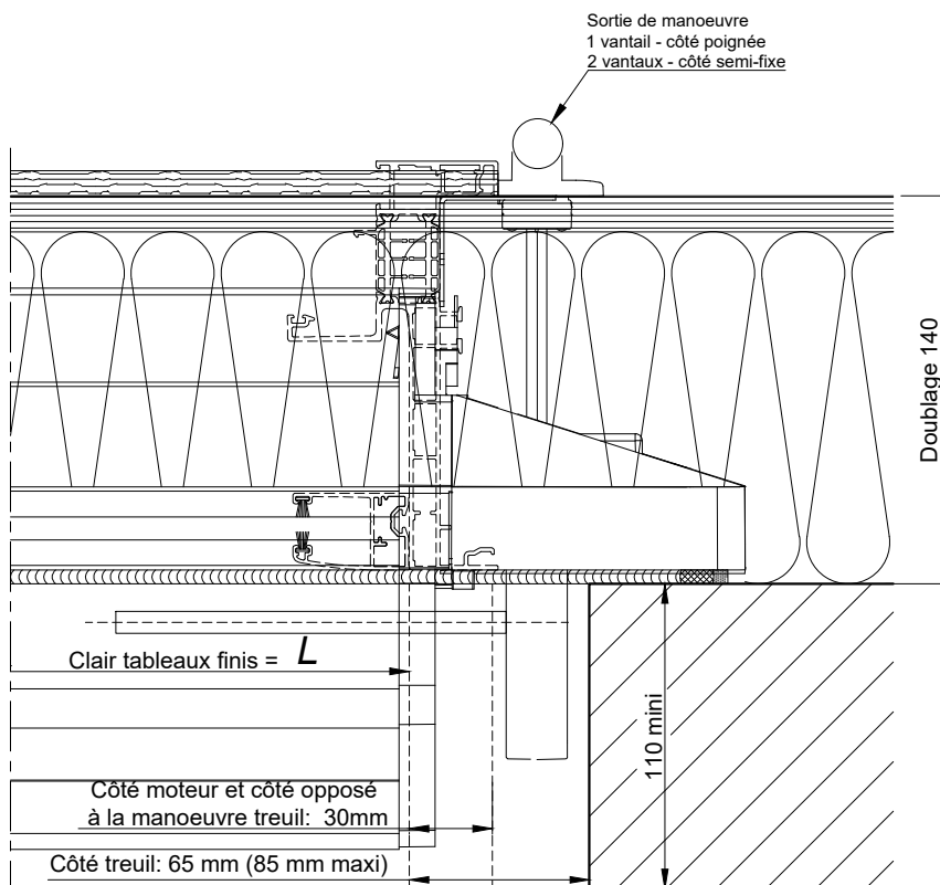
COUPE HORIZONTALE Ech 1/3
