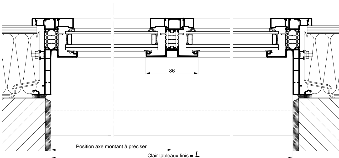
COUPE HORIZONTALE Ech 1/3
