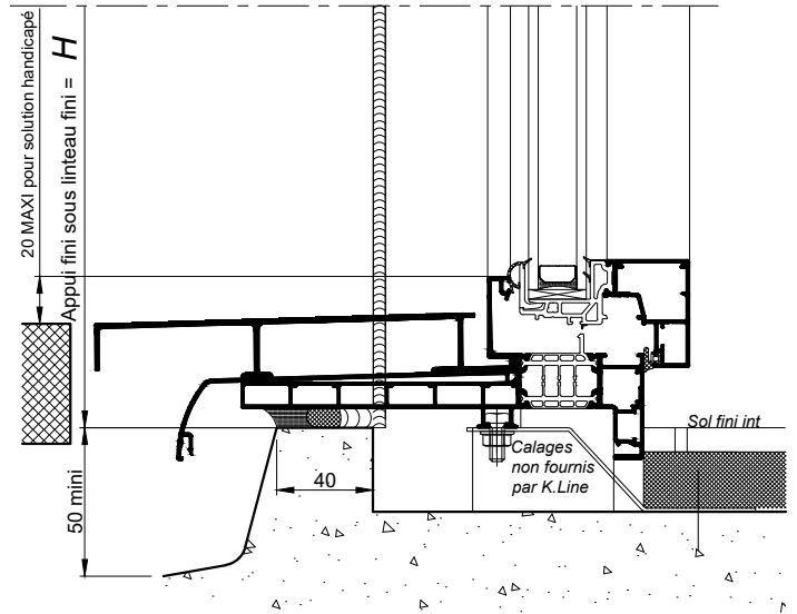
DOUBLAGE DE 120 - Appui déporté
