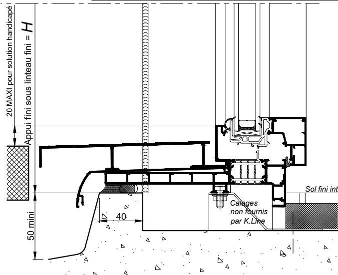
DOUBLAGE DE 120 - Appui non déporté
