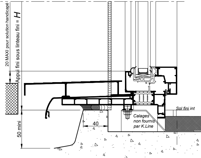
DOUBLAGE DE 120 - Appui non déporté
