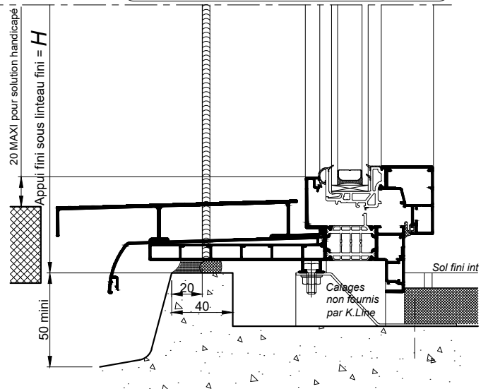
DOUBLAGE DE 120 - Appui déporté
