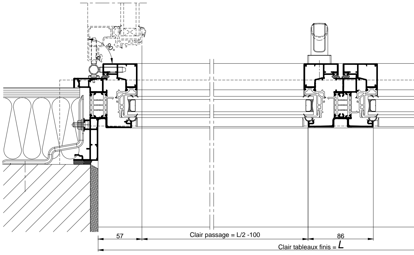
COUPE HORIZONTALE PARTIELLE Ech 1/3
