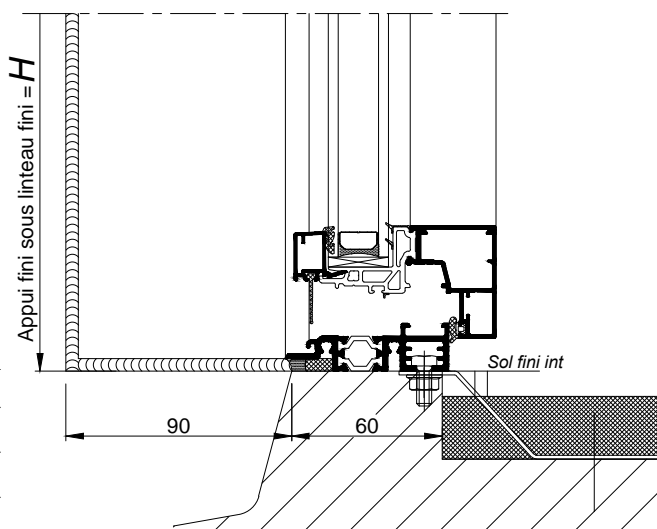
COUPE VERTICALE PARTIELLE Ech 1/3
