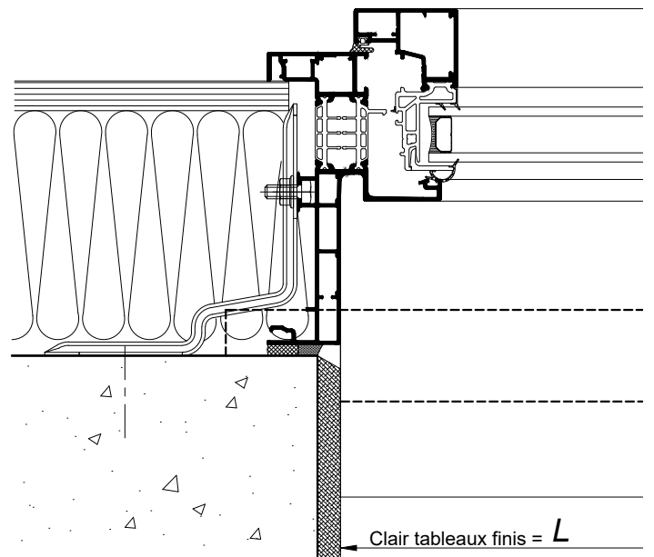
COUPE HORIZONTALE Ech 1/3
