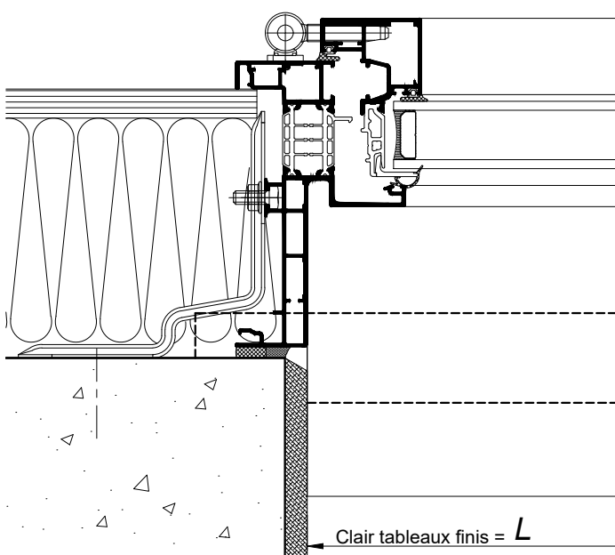
COUPE HORIZONTALE Ech 1/3
