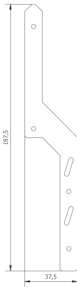
GOUSSET GALANDAGE : 11226899
