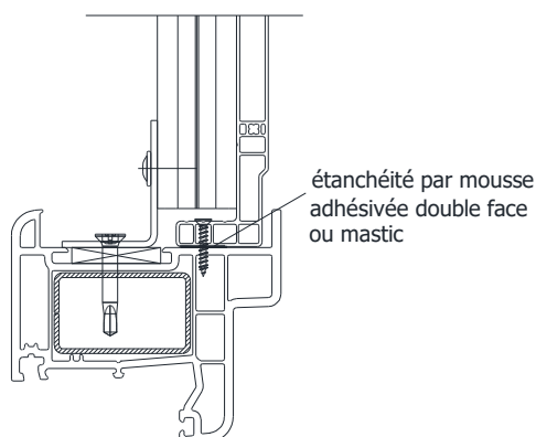
Doublage 120 mm
