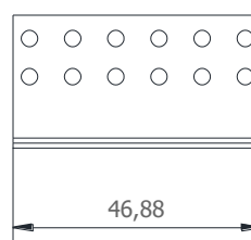
EQUERRE GALANDAGE : 11226999
