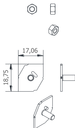
CLAMEAU + ECROU 6 : 11148499
