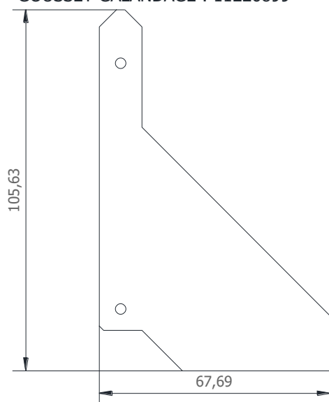
GOUSSET GALANDAGE : 11226899
