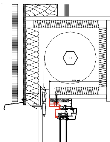
Caisson menuisé
